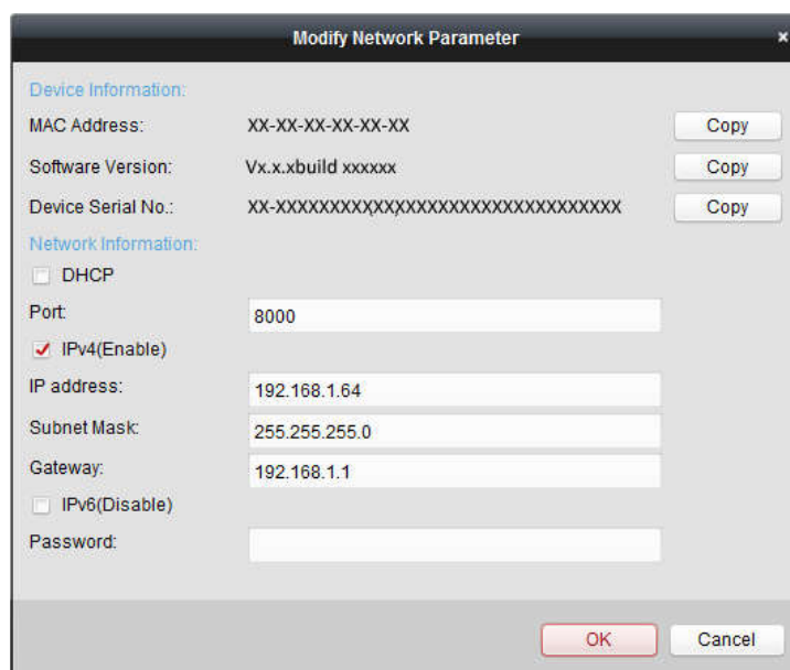
Рисунок 2-9 Меню изменения сетевых параметров
